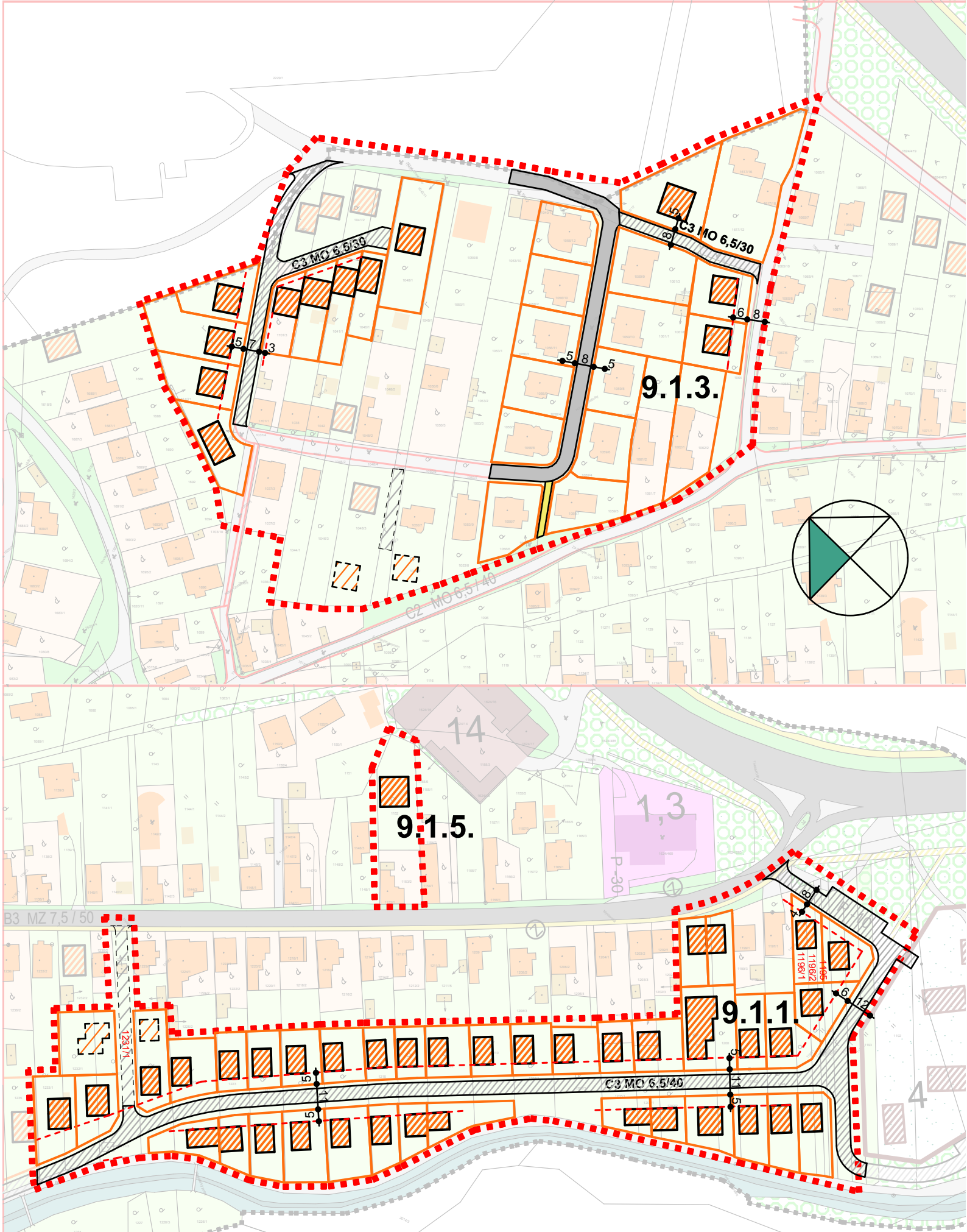
ZMENY A DOPLNKY ÚPN-Z MYSLAVA 2011 výkres č.2 KOMPLEXNÝ NÁVRH, DOPRAVA M=1:2000 LOKALITY 9.1.1., 9.1.3., 9.1.5.
