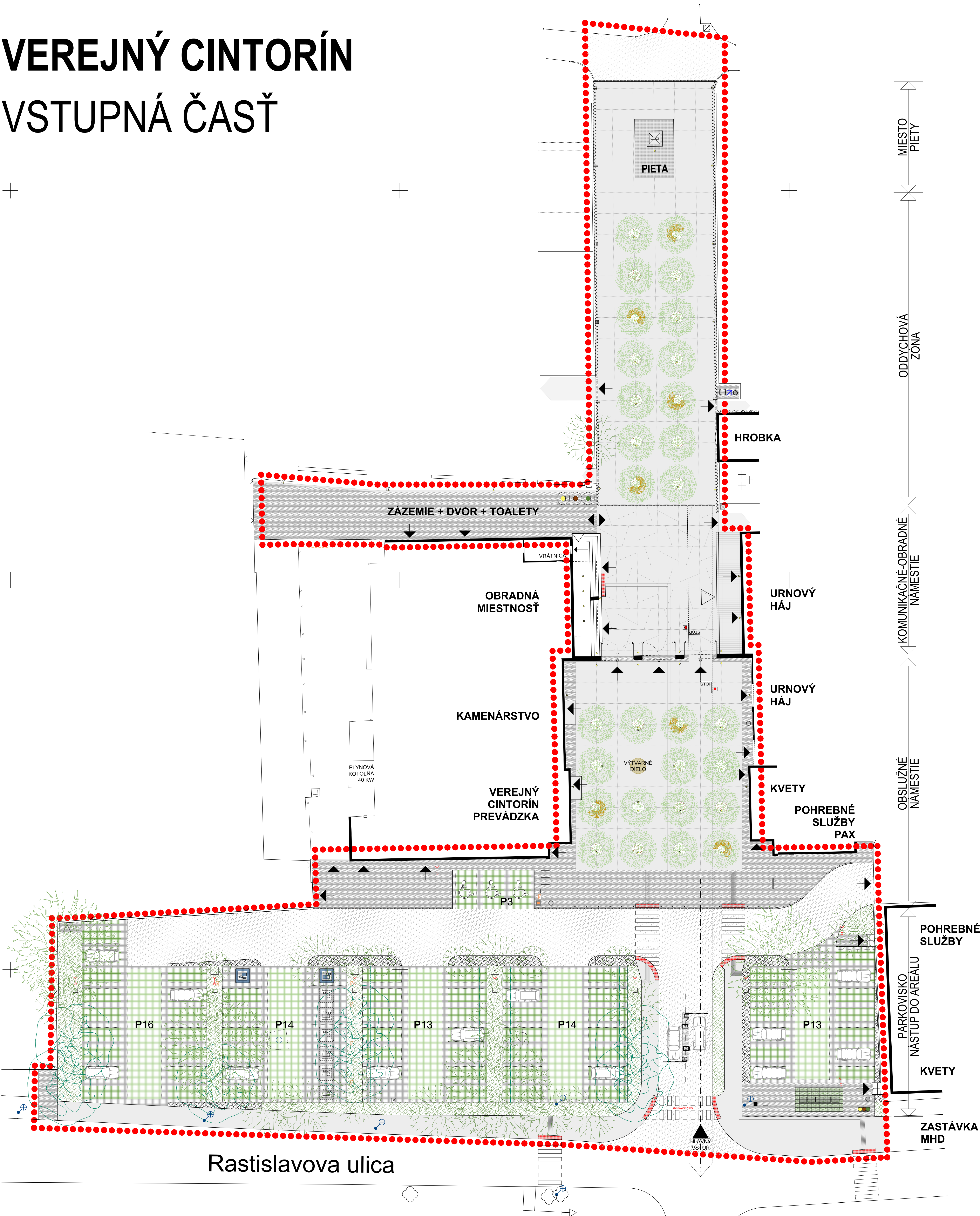
ZASTAVOVACIA SITUÁCIA STAVBY M 1:200
