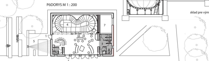
PŔDORYS M 1 : 200
